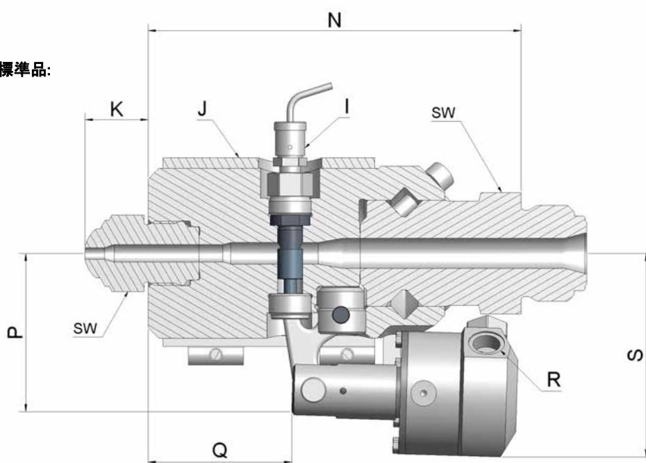
標準的な寸法 (mm)
